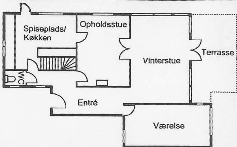
1. Sal
